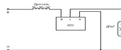
Рис. 2 Схема включения
